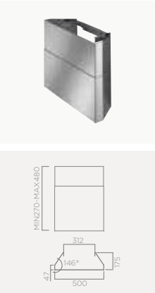
Zestaw opcjonalny Komin KAE CX
